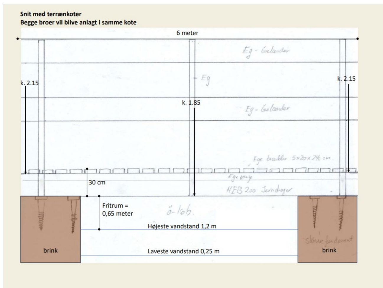
Figur 4. Principskitse over broernes udformning
